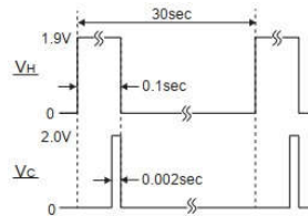
타이밍 차트
